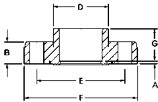
Flange Van Stone Style Loose Ring Soc
