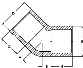
45° Elbow Soc x Soc
