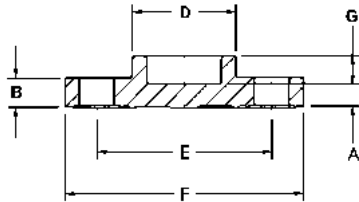
Flange Blind Soc
